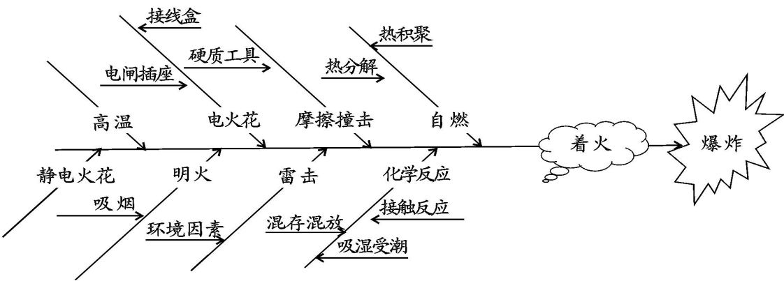
图 3-1 烟花爆竹引爆的因果分析图
